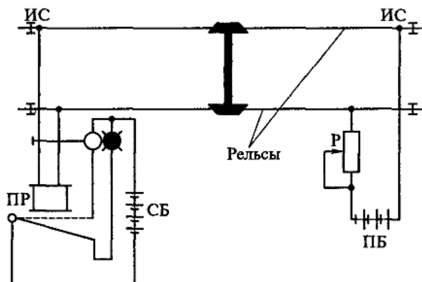
Схема двужначной автоматической блокировки:
