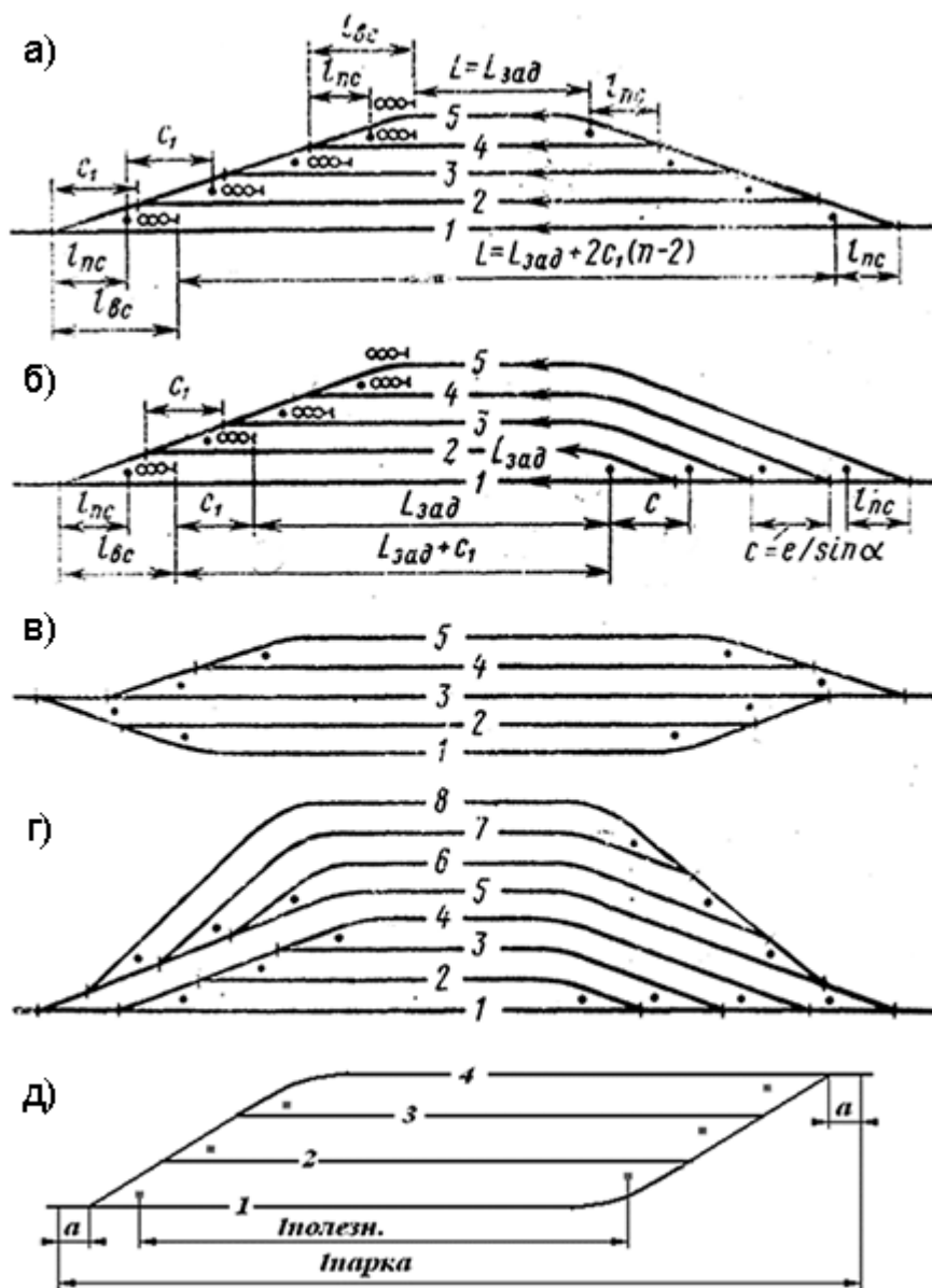
Рис. 1 – Основные схемы железнодорожных парков путей: а – схема трапециевидального парка; б – схема парка «трапециев»; в – схема парка «рыбка»; г – схема комбинированного парка; д – схема парка параллелограмма
