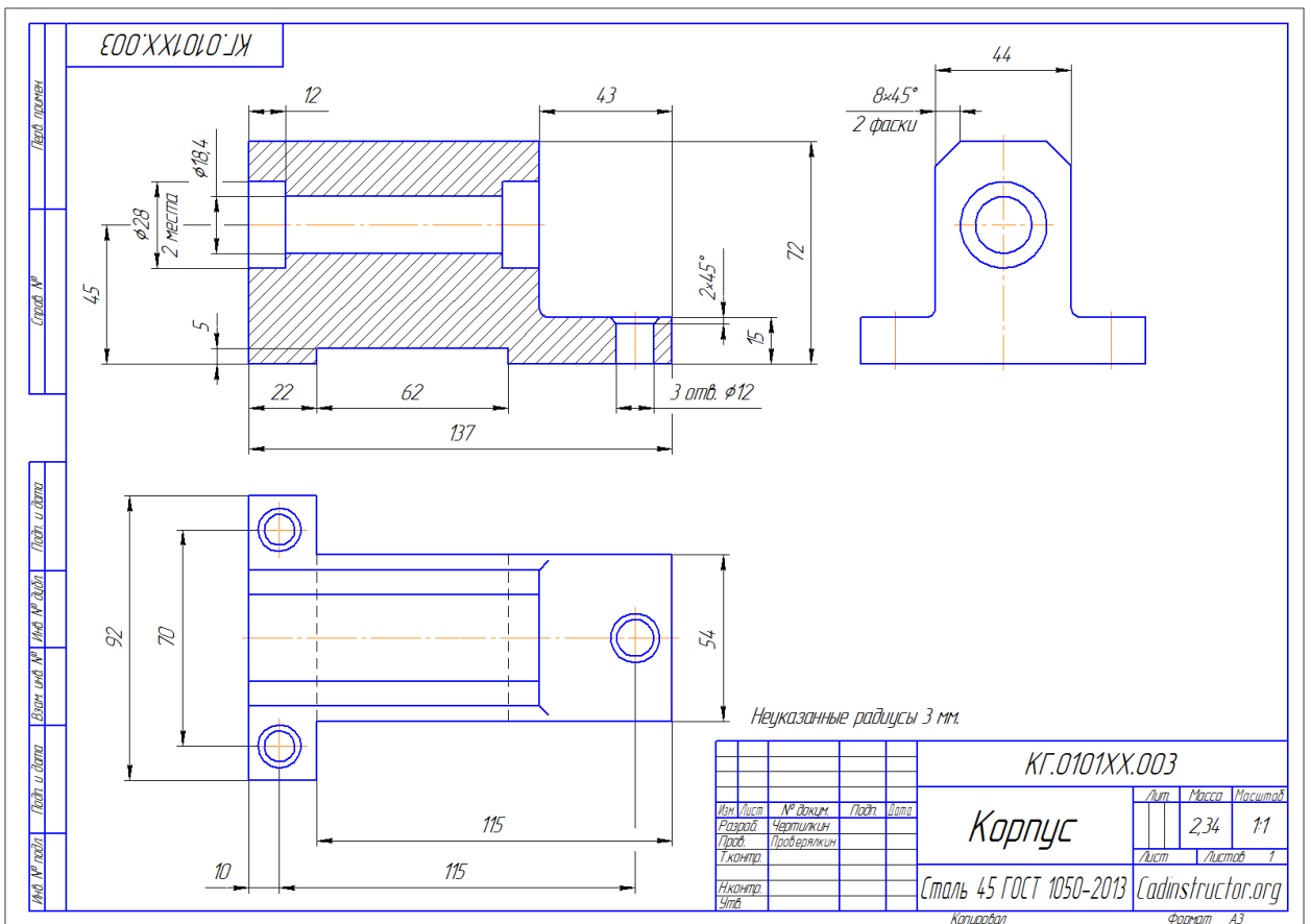
Пример выполнения графической работы №6 «Построение простого разреза»
