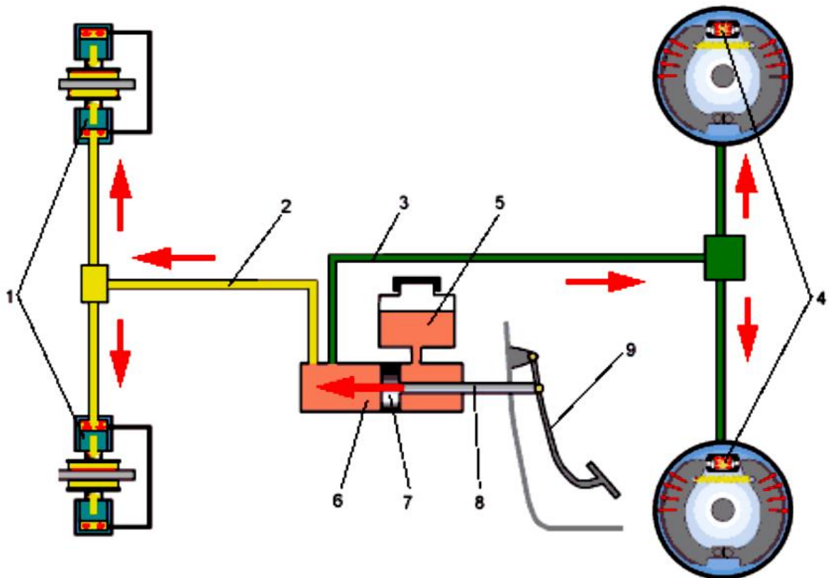
Рисунок 14.1 – Схема рабочей тормозной системы легкового автомобиля
