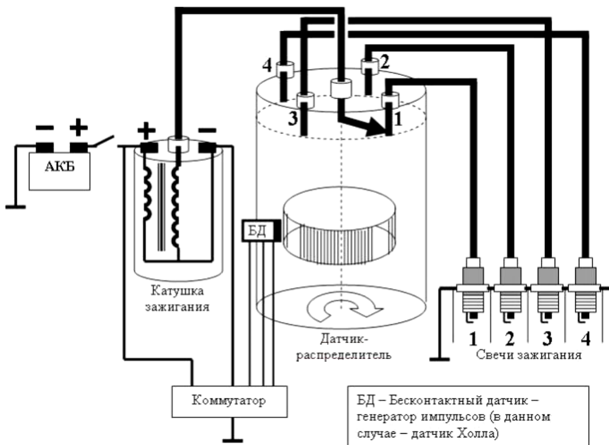
Рисунок 8.1 – Схема бесконтактной системы зажигания
